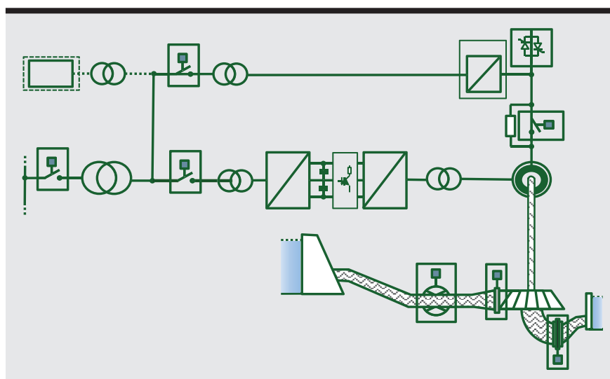
Bild 4 Schematischer Aufbau einer Anlage mit Vollumrichter.
